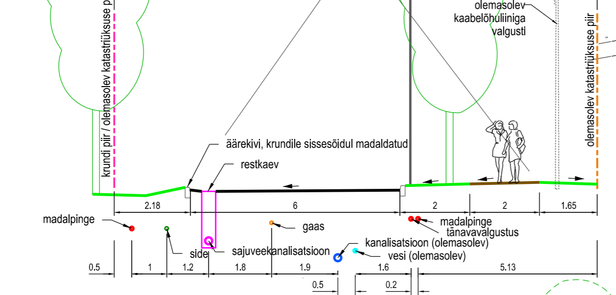
HIPODROOMI TÄNAVA LÕIGE 2-2
