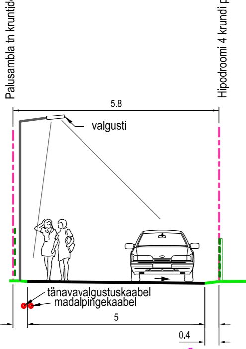
PALUSAMBLA TN KRUNTIDE JA HIPODROOMI 4 KRUNDI VAHELINE TEE LÕIGE 3-3
