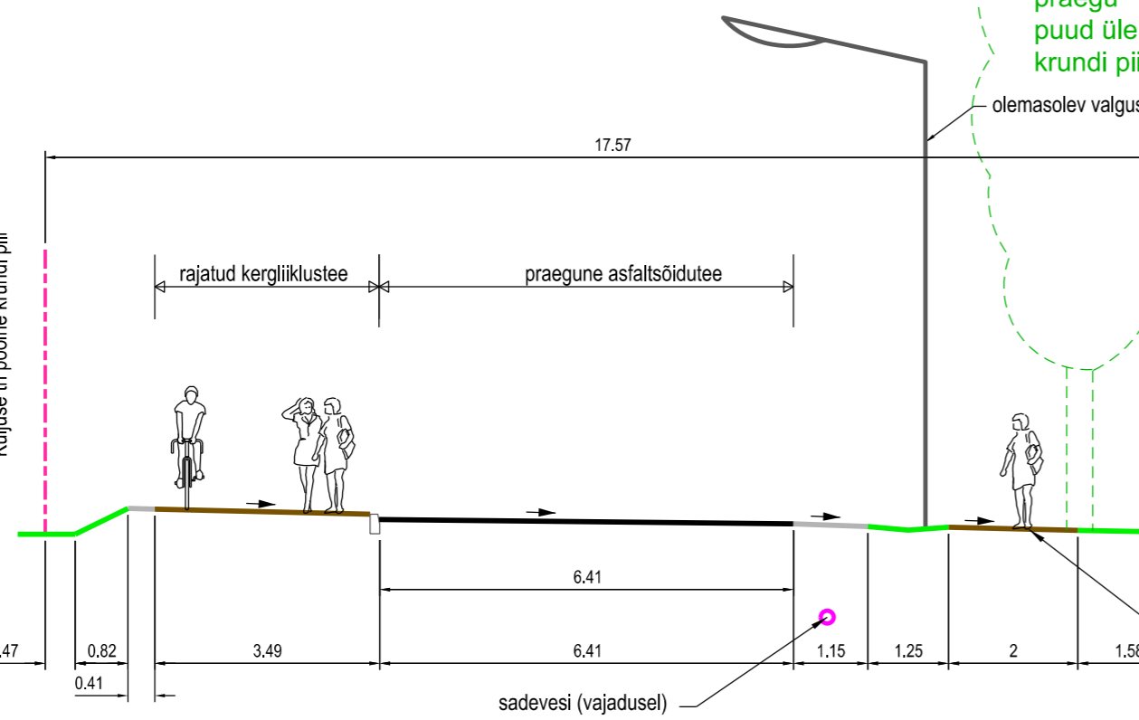
HIPODROOMI TÄNAVA LÕIGE 2-2
