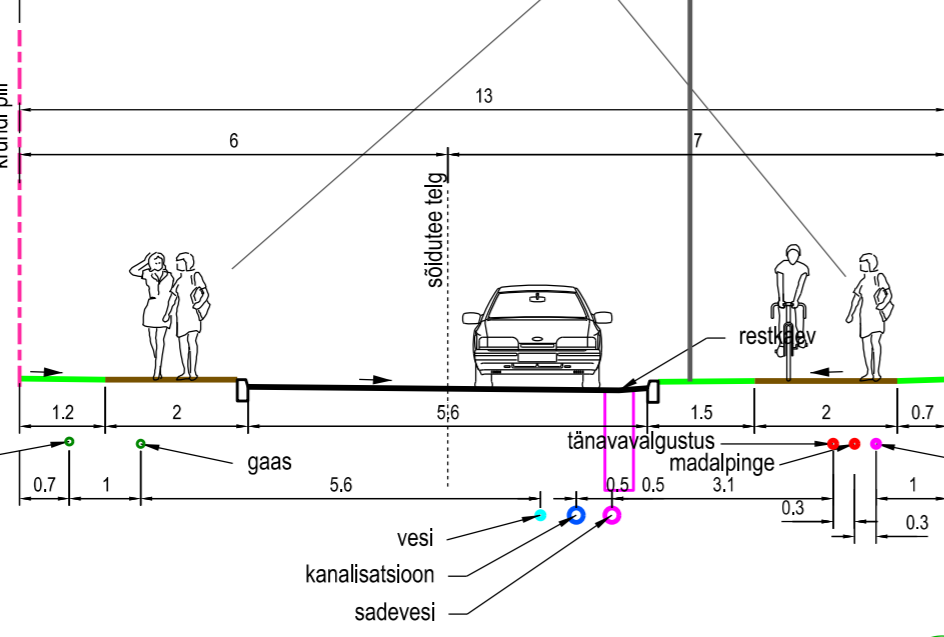
PLANEERITUD TÄNAVA LÕIGE 1-1
